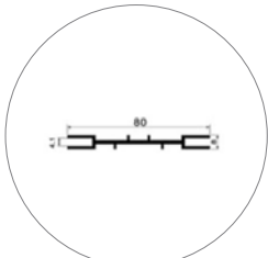
CABO-80-SEG 165.9" W (qty 4)
