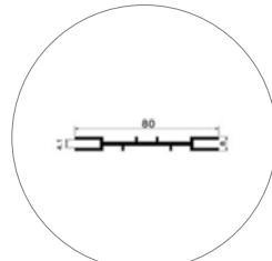
CABO-80-SEG 74.7 W (qty 8)
